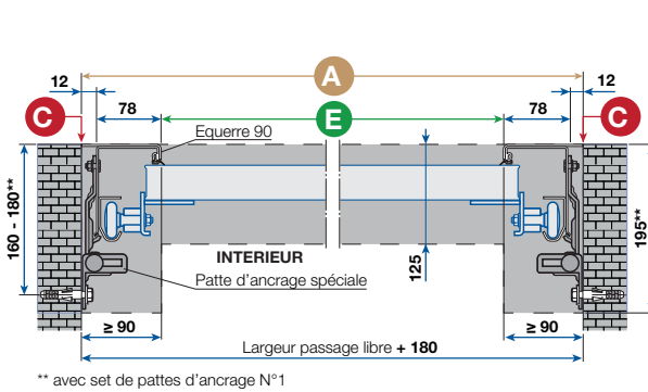
Coupe en largeur - Porte avec pattes d'ancrage spéciales
