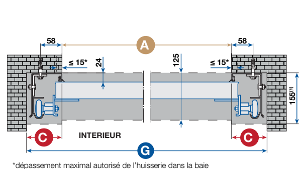
Coupe en largeur - Porte livrée en kit
