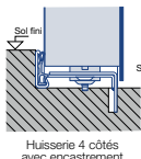
Huisserie 4 côtés avec encastrement au sol
