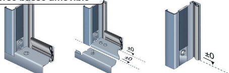
Huisserie 4 côtés avec encastrement au sol
