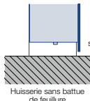
Huisserie sans battue de feuillure en traverse basse
