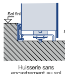
Huisserie sans encastrement au sol
